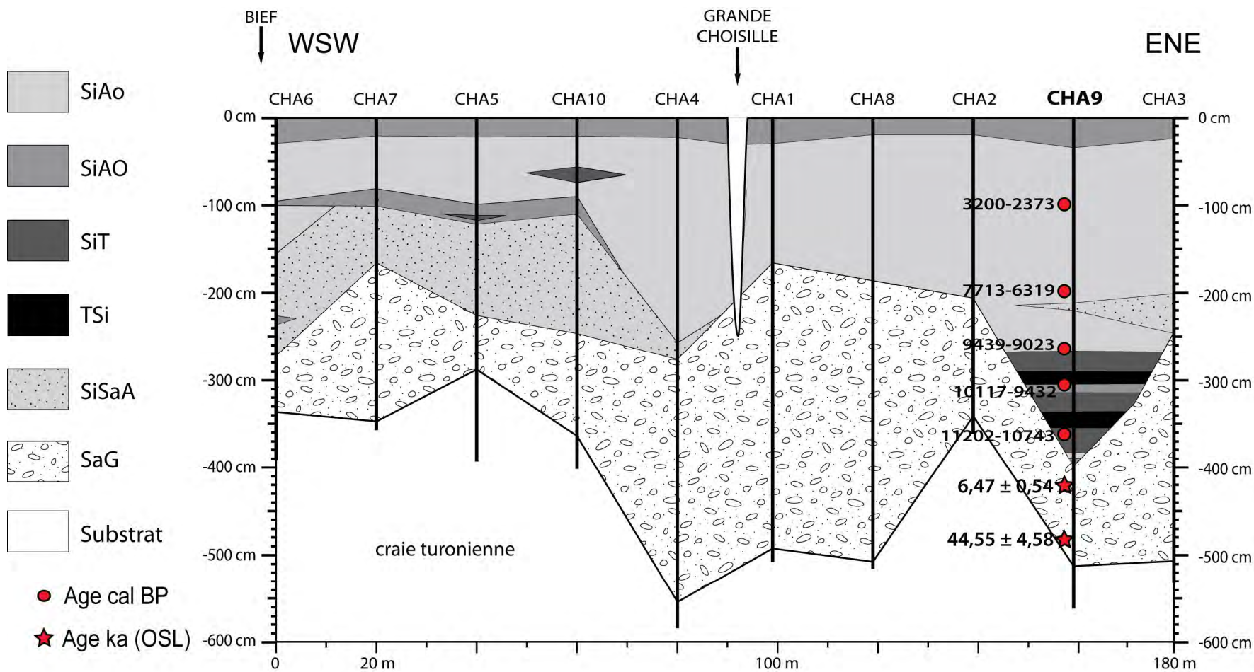
Figure 2.45 : transect lithologique sur le site CHA
