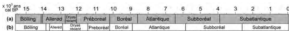
Figure 2.4 : comparaison des chronozones régionaux et conventionnelles.
