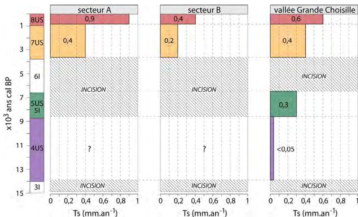
Figure 7.13 : valeurs des taux de sédimentation moyens (Ts en mm.an -1 ) dans les secteurs A et B et dans la vallée principale de la Grande Choissille (incluant les secteurs C et D)
