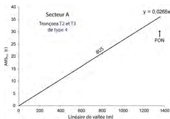
Figure 7.6 : régressions linéaires appliquées au calcul d' AMS_{tron} pour 8US dans les tronçons de classe 4
