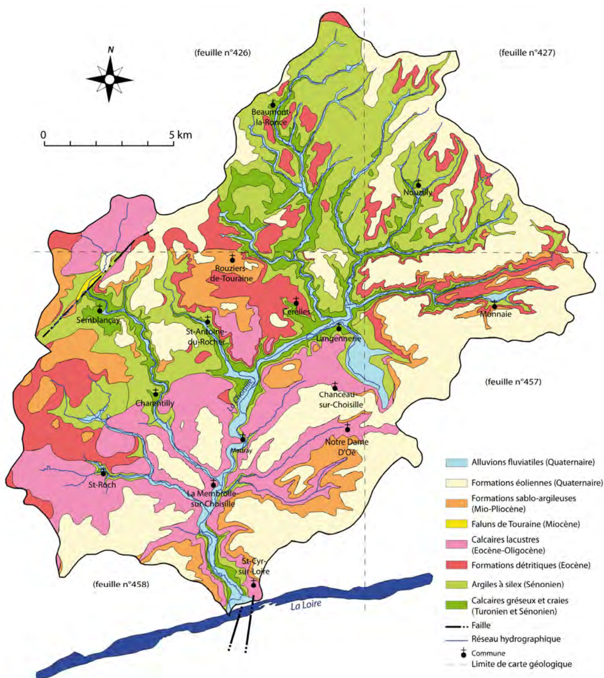
Figure 1.7 : carte géologique simplifiée du bassin versant de la Choisille (modifié d'après Alcaydé, 1968 ; Rasplus et al., 1974 ; Manivit et al., 1975 ; Manivit et al., 1998)
