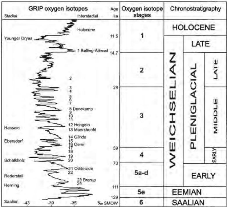
Figure 6.1 : chronostratigraphie du Quaternaire récent et comparaisons avec l'enregistrement \delta^{18}\text{O} de la carotte GRIP (Johnsen et al. , 1992), les stades isotopiques de l'oxygène des sédiments marins (Martinson et al. , 1987), et les interstades et stades continentaux de l'Europe du nord-ouest (d'après Bos et al. , 2001)
