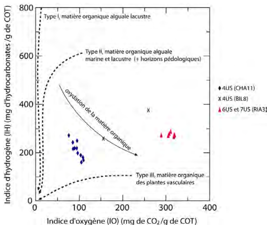
Figure 5.2 : diagramme de Van Krevelen de type IH-IO appliqué à la matière organique sédimentaire des échantillons de faciès SiT ou TSi (modifié d'après Espitalié et al. , 1985 et Meyers et Lallier-Vergès, 1999). Pour la matière organique de type I, II et III, le chemin d'altération thermique du matériau source vers le graphite (100 % de COT) est indiqué en tirets. Le chemin d'altération par oxydation depuis les matériaux de types I et II jusqu'à ceux de type III est indiqué en trait plein
