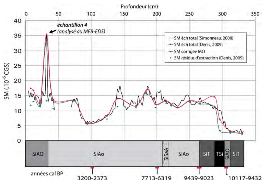
Figure 3.22 : susceptibilité magnétique le long de la carotte CHA9 (modifié d'après Simmoneau, 2008 ; Denis, 2009)
