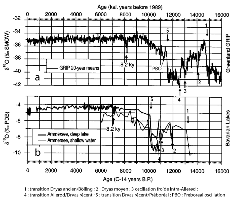
Figure 6.3 : moyennes pluri-décennales (20 ans) des valeurs de \delta^{18}\text{O} (a) du GRIP (Summit, Groenland) et (b) des ostracodes du lac Ammersee (Allemagne) depuis 16000 ans (modifié d'après von Grafenstein et al. , 1998)
