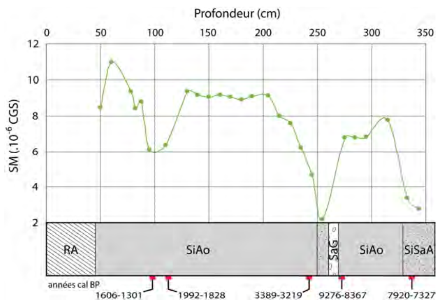
Figure 3.21 : susceptibilité magnétique le long du forage BJE9 (modifié d'après Denis, 2009)
