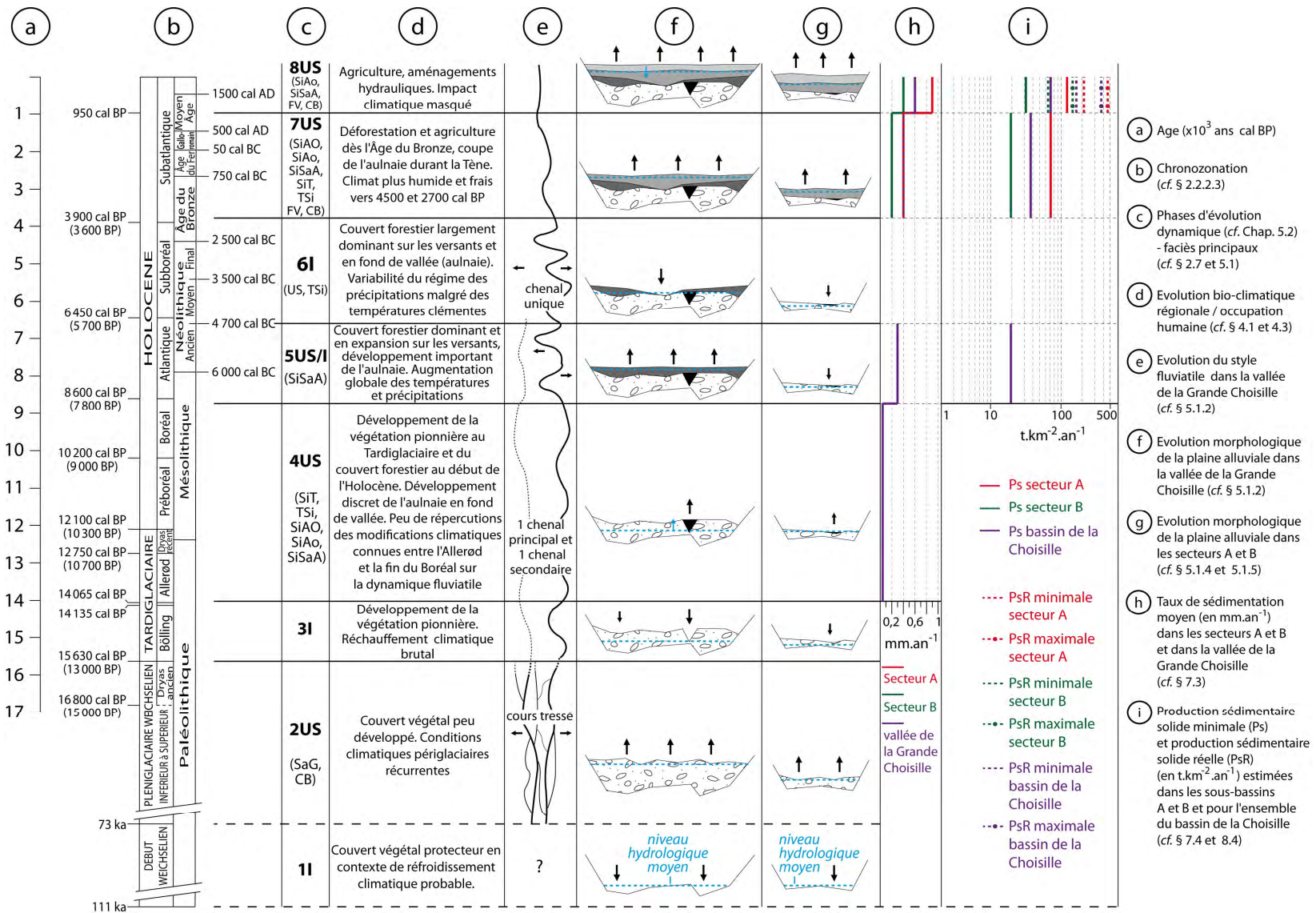
Figure 8.1 : synthèse de l'évolution du bassin de la Choisille depuis le Weichsélien
