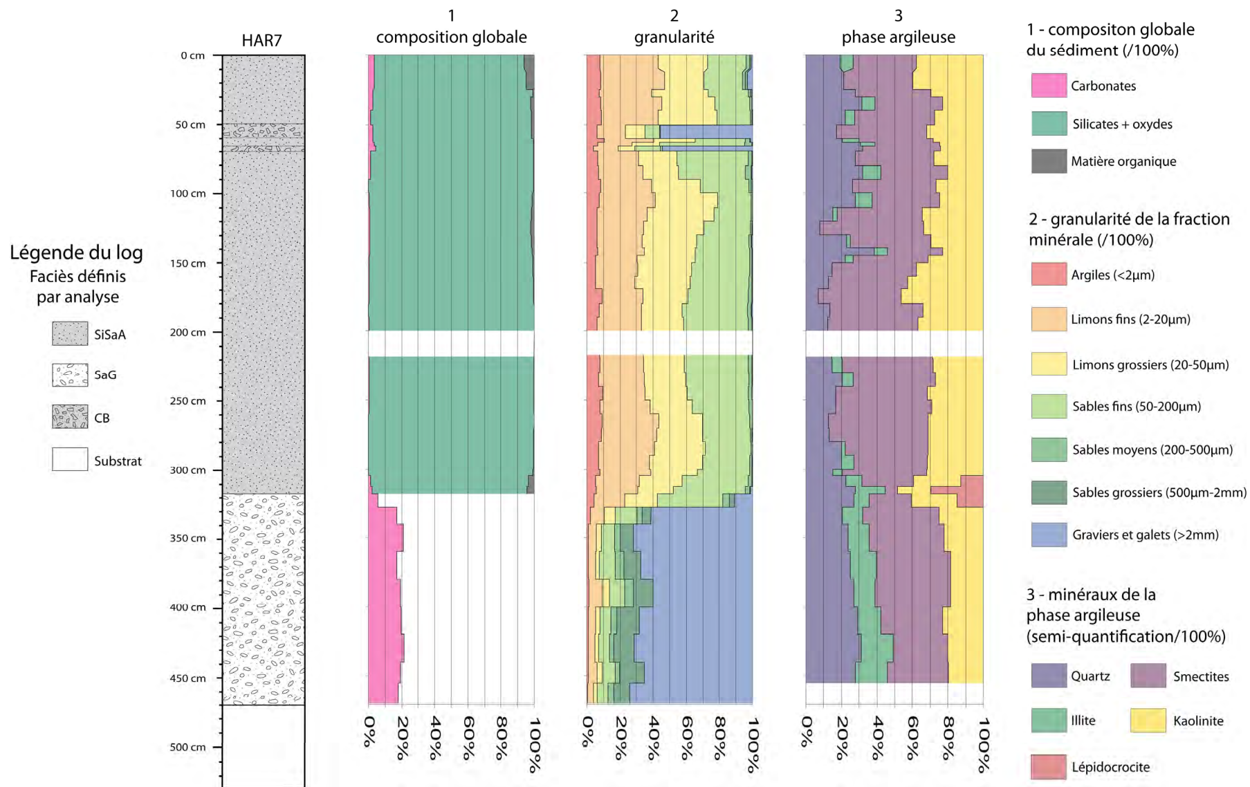
Figure 2.15 : résultats des analyses dans le forage HAR7
