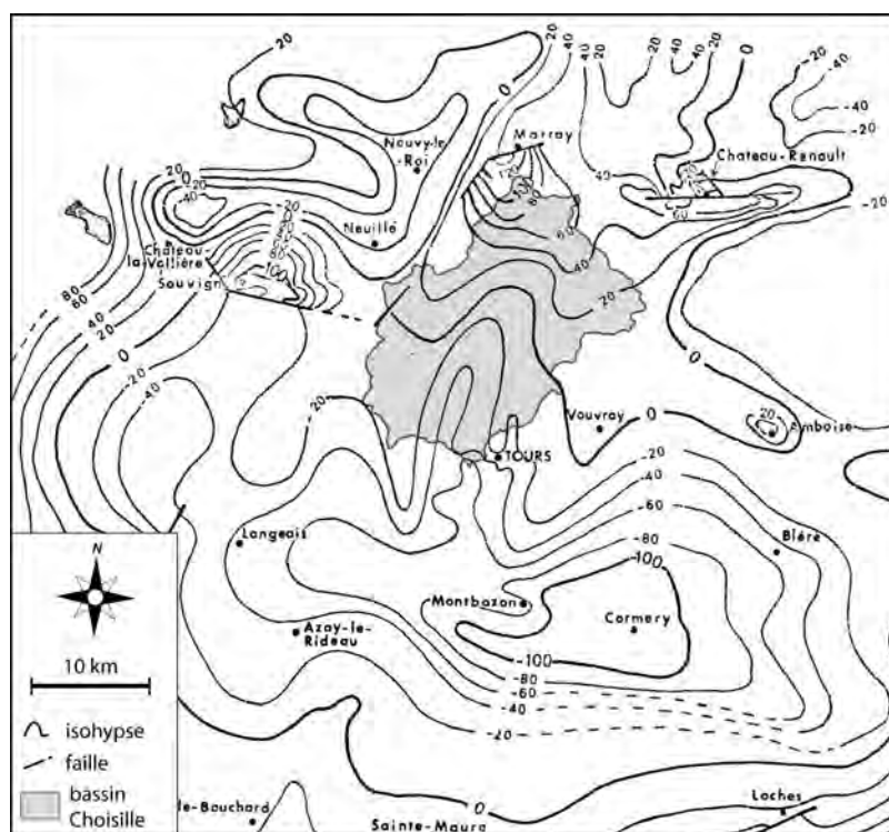
Figure 1.4 : carte des isohypses du toit du Cénomanien dans les environs du bassin de la Choisille (modifié d'après Rasplus, 1978)
