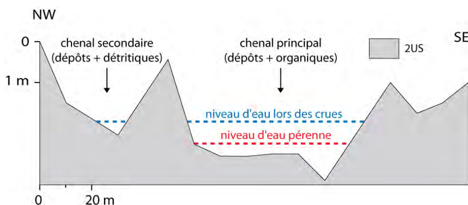
Figure 5.5 : représentation schématique montrant les niveaux d'eau relatifs entre le chenal principal et le chenal secondaire durant l'Allerød sur le transect BRO
