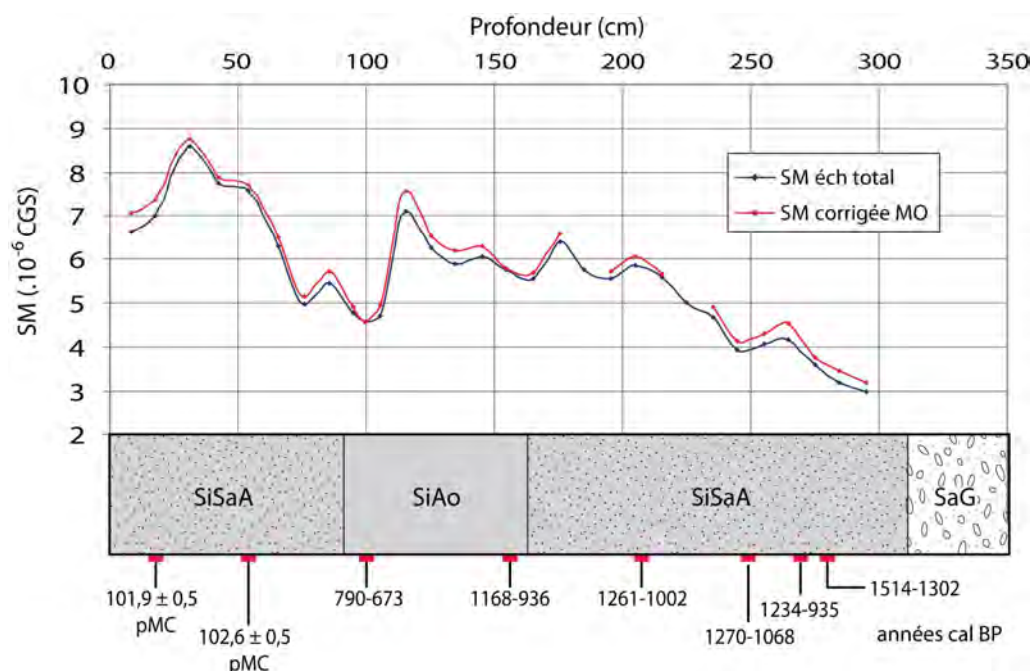
Figure 3.20 : susceptibilité magnétique le long du forage NAU1 (modifié d'après Denis, 2009)
