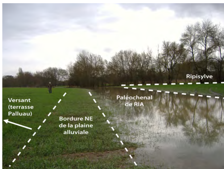
Figure 5.3 : photographie d'une décrue de la Choisille le 13 février 2007 sur le site RIA, en rive gauche (cliché F. Hinschberger). Le paléochenal de RIA, point bas dans la plaine alluviale, est en eau
