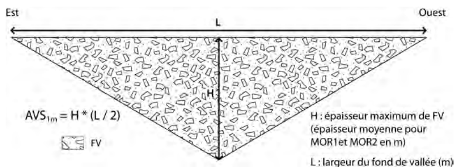
Figure 7.2 : méthode de calcul d' AVS_{Im} sur le site MOR (secteur A)
