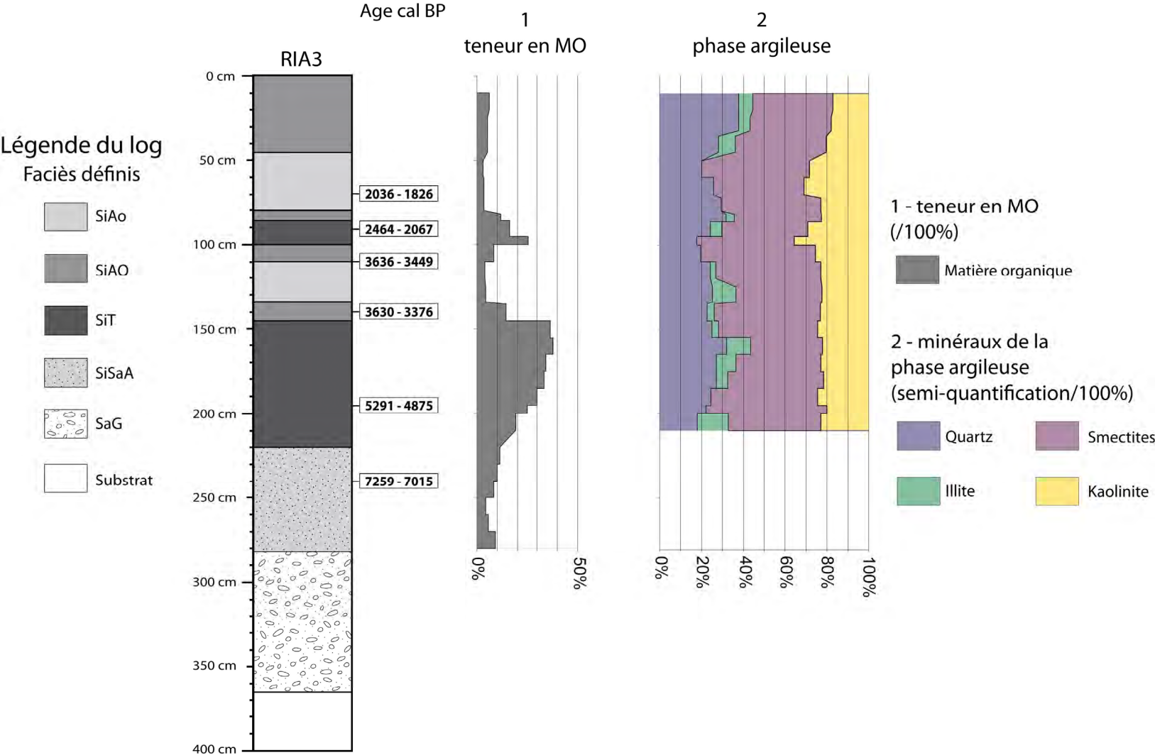
Figure 2.49 : résultats des analyses dans le forage RIA3
