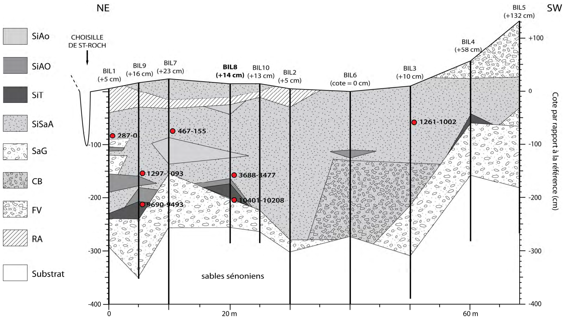
Figure 2.32 : transect lithologique sur le site BIL
