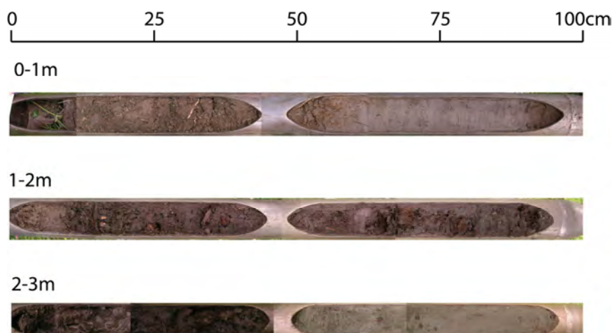
Figure 2.23 : photographie de la carotte ROC3 entre 0 et 3 m de profondeur
