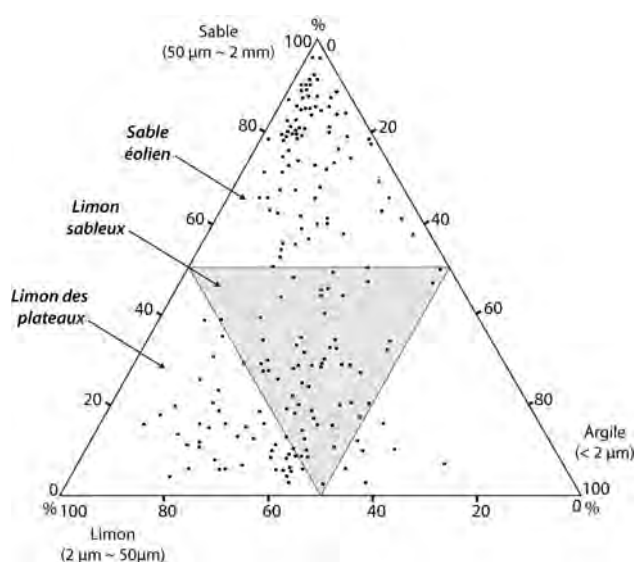
Figure 1.10 : granularité des sédiments éoliens de Touraine (modifié d'après Macaire, 1986a)
