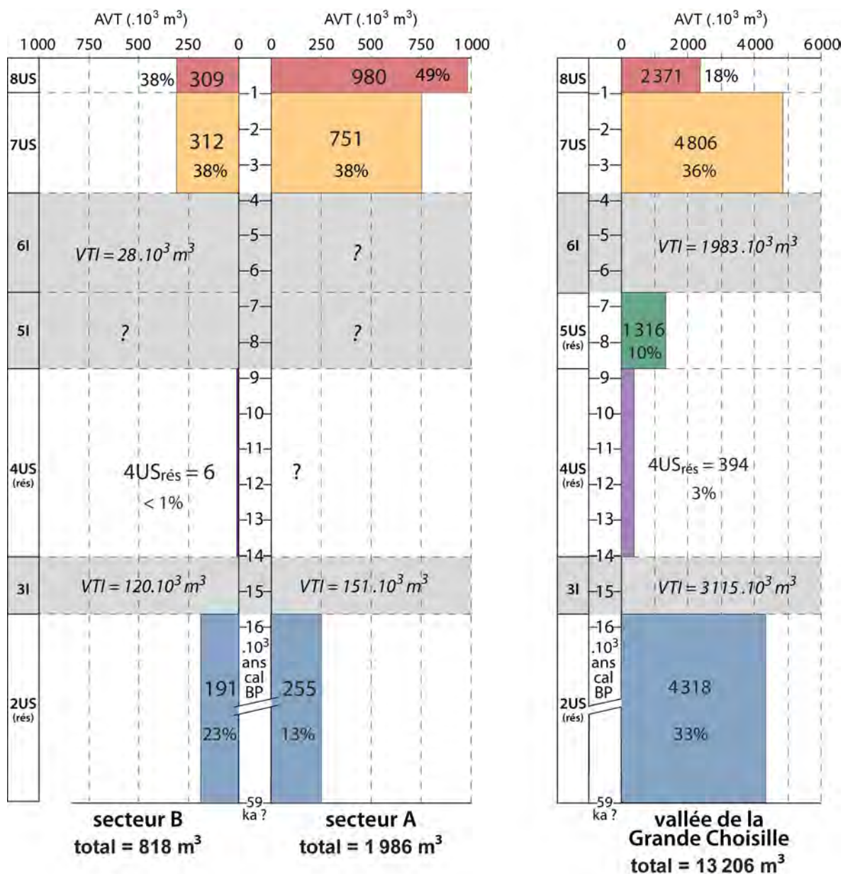
Figure 7.12 : valeurs d'accumulation volumique totale (AVT en \cdot 10^3 \text{ m}^3 ) et de volume total incisé (VTI en \cdot 10^3 \text{ m}^3 ) pour chaque phase dans les secteurs A et B et dans la vallée de la Grande Choissille (incluant C et D)
