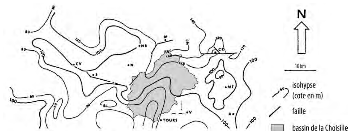
Figure 1.6 : carte des isohypse du mur de l'Eocène dans les environs du bassin de la Choisille (modifié d'après Rasplus, 1978)
