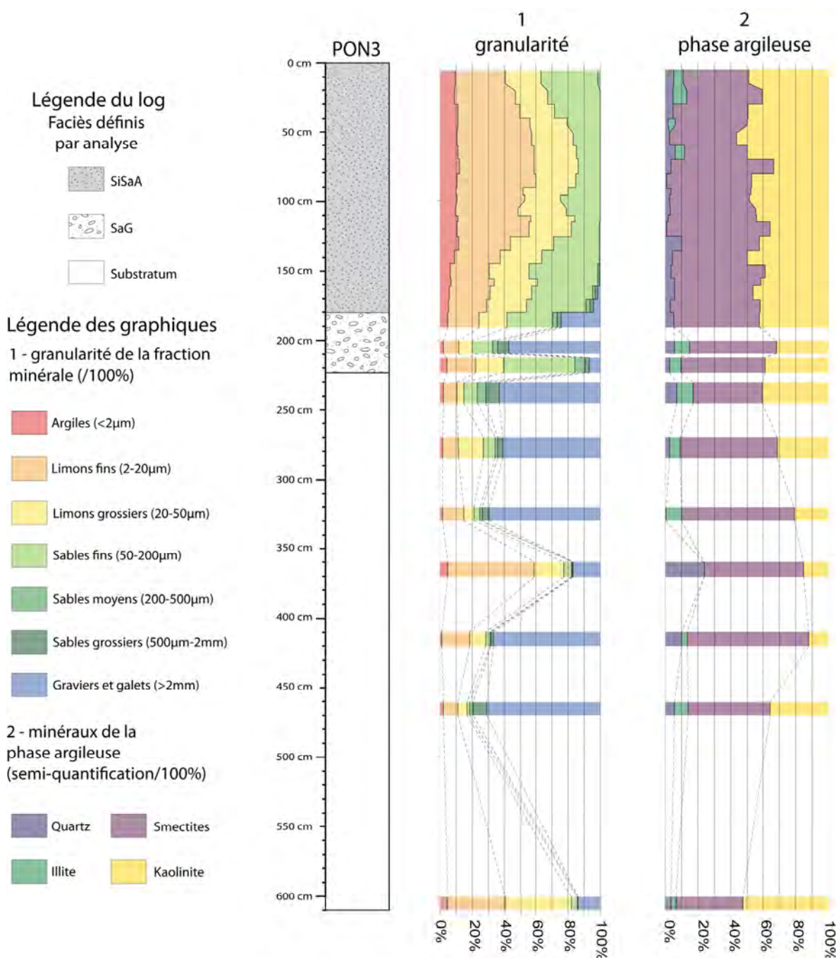
Figure 2.7 : résultats des analyses dans le forage PON3
